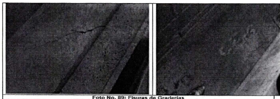
Foto No. 89: Fisuras de Graderías
